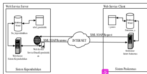
Gambar 3. Arsitektur Integrasi Web Services antara Sistem Kependudukan dengan Sistem Puskesmas
