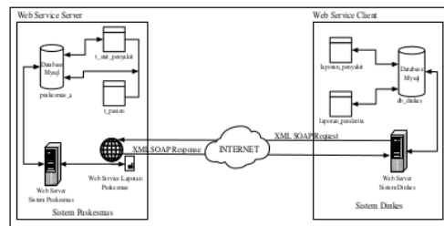
Gambar 5 Arsitektur Integrasi Web Services Sistem Puskesmas dengan Sistem Dinas Kesehatan
