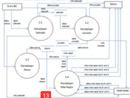
Gambar 8. DFD Level 1 proses pendataan
