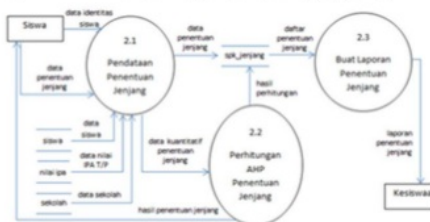
Gambar 9. DFD Level 1 penentuan jenjang
