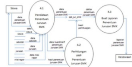
Gambar 11. DFD Level 1 penentuan jurusan
