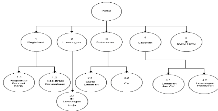
Gambar 2 Dekomposisi Diagram
