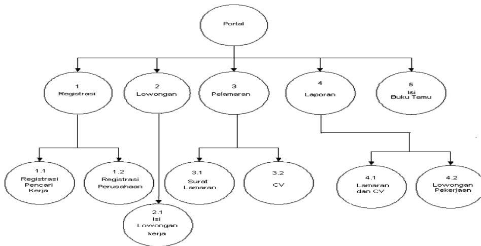
Gambar 2 Dekomposisi Diagram
