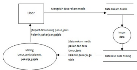
Gambar 2. DFD level 1
