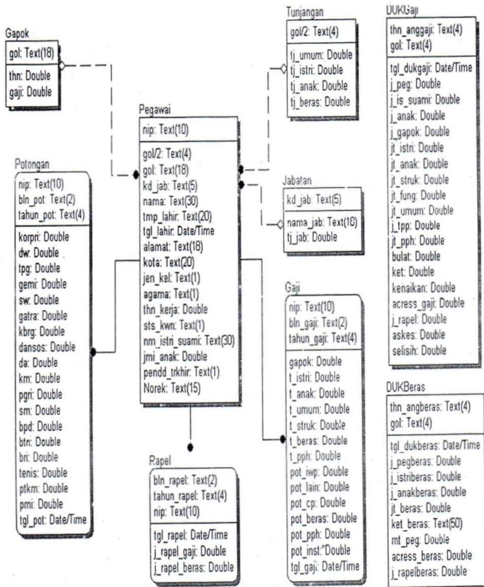
Gambar 2: Relasi Antar Tabel
