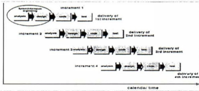
Gambar 2.1: Pengembangan Sistem Model Incremental
