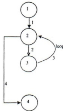
Gambar 5.4: Grafik Alir Proses Ambil Data Pegawai
