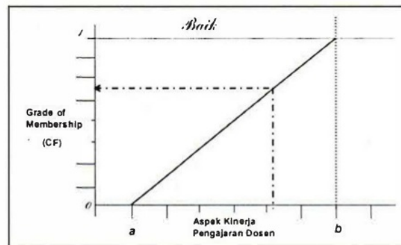
Gambar 2. Representasi Himpunan Fuzzy Baik
