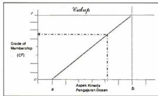
Gambar 3. Representasi Himpunan Fuzzy Cukup
