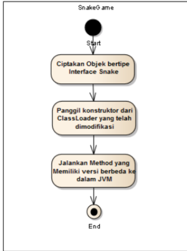
Gambar 4 Diagram Aktifitas Memuat Kelas ke dalam JVM
