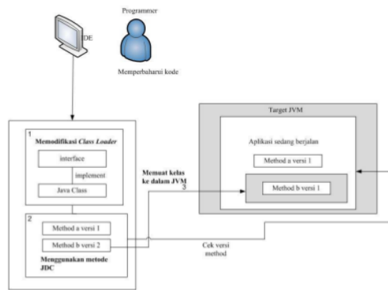
Gambar 1 Metode yang Diusulkan
