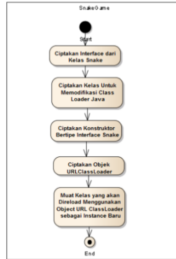
Gambar 2 Diagram Aktifitas Memodifikasi ClassLoader
