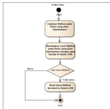
Gambar 3 Diagram Aktifitas Penggunaan Metode JDC
