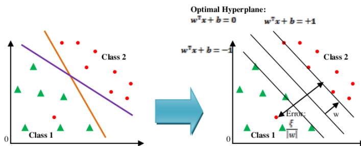
Gambar 1. Mencari fungsi pemisah (hyperplane) secara linier
