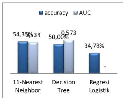
Gambar 2. Perbandingan kinerja model individu
