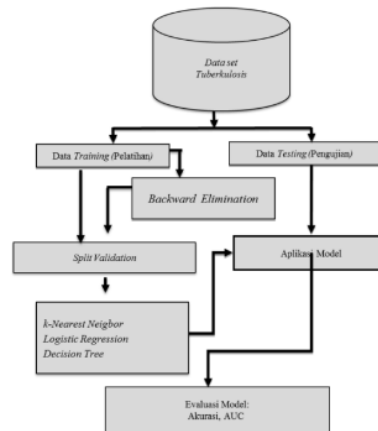
Gambar 1. Diagram Alir Eksperimen
