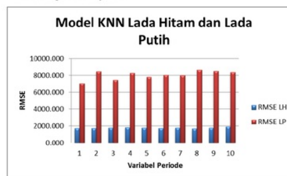
Gambar 3 Grafik Kinerja Model KNN untuk Lada Hitam dan Lada Putih
