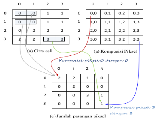
Gambar 2. Penentuan awal matrik bebas pasangan dua piksel
