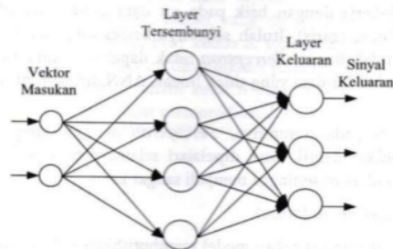
Gambar 3. Arsitektur Backpropagation [13]
