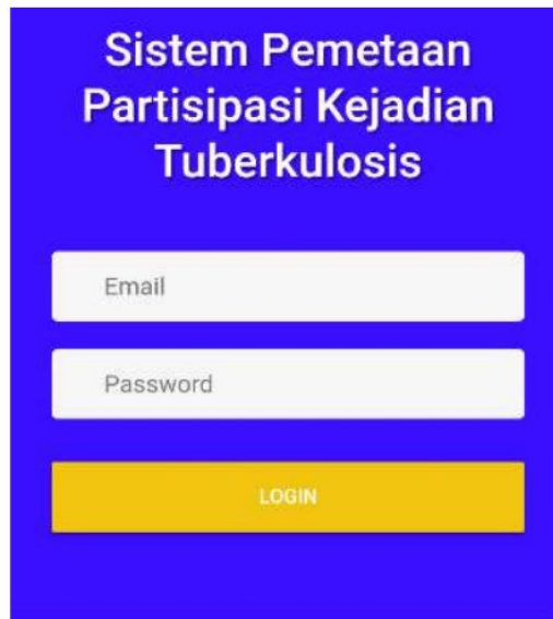
Gambar 1. Halaman Login
