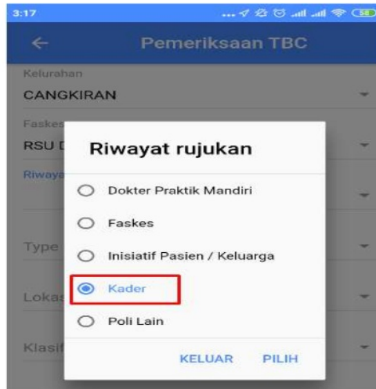
Gambar 18. Riwayat Rujukan
