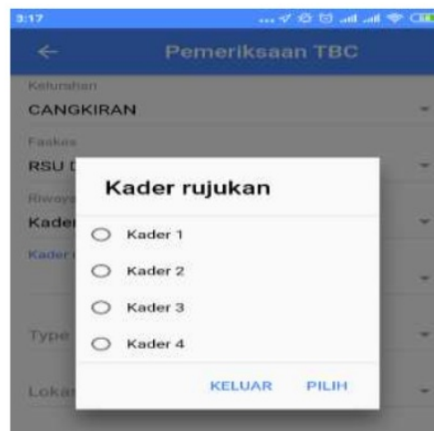
Gambar 19 Kader Rujukan
