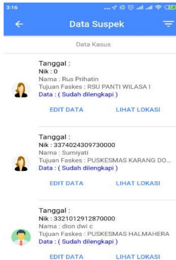
Gambar 12. Data Suspek
