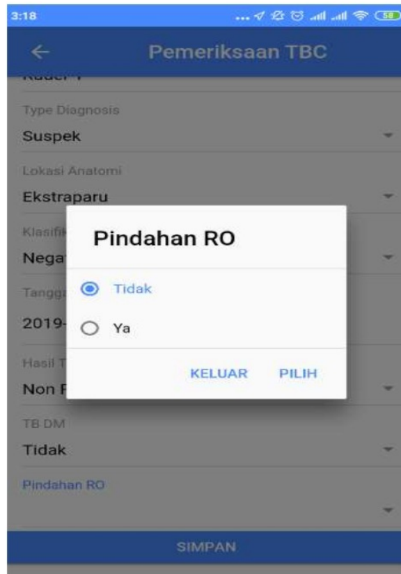
Gambar 26. Pindahan RO
