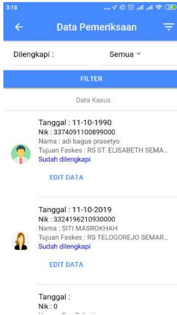
Gambar 27. Data Pemeriksaan
