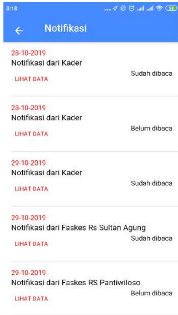
Gambar 28.List Notifikasi
