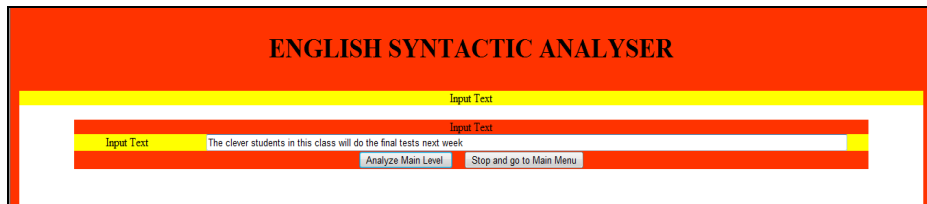
Gambar 3. Input text
