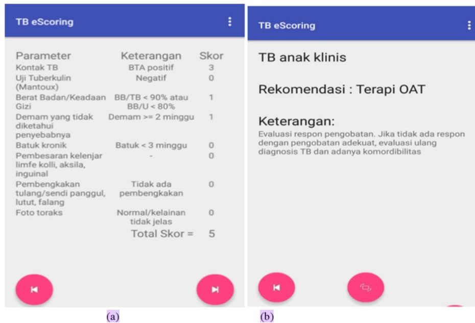
Gambar 6. Tampilan menu hasil penilaian (a) Ringkasan perhitungan skor dan (b) Rekomendasi tindakan dari diagnosis
