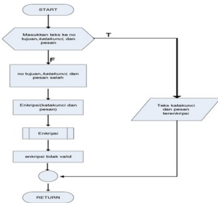
Gambar 6. Gambar proses enkripsi
