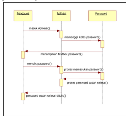
Gambar 3. Diagram pemakaian password
