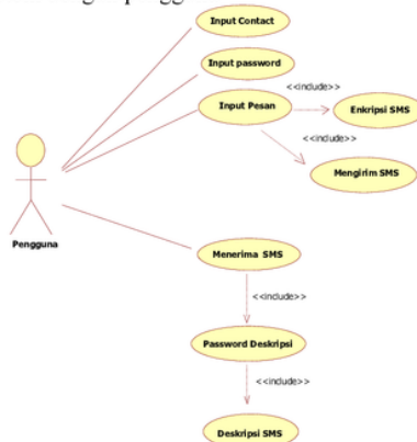
Gambar 2. Interaksi Sistem Dengan User
