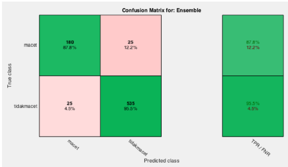
Gambar 9. Eksperimen 4.4.5 : Confusion Matrix
