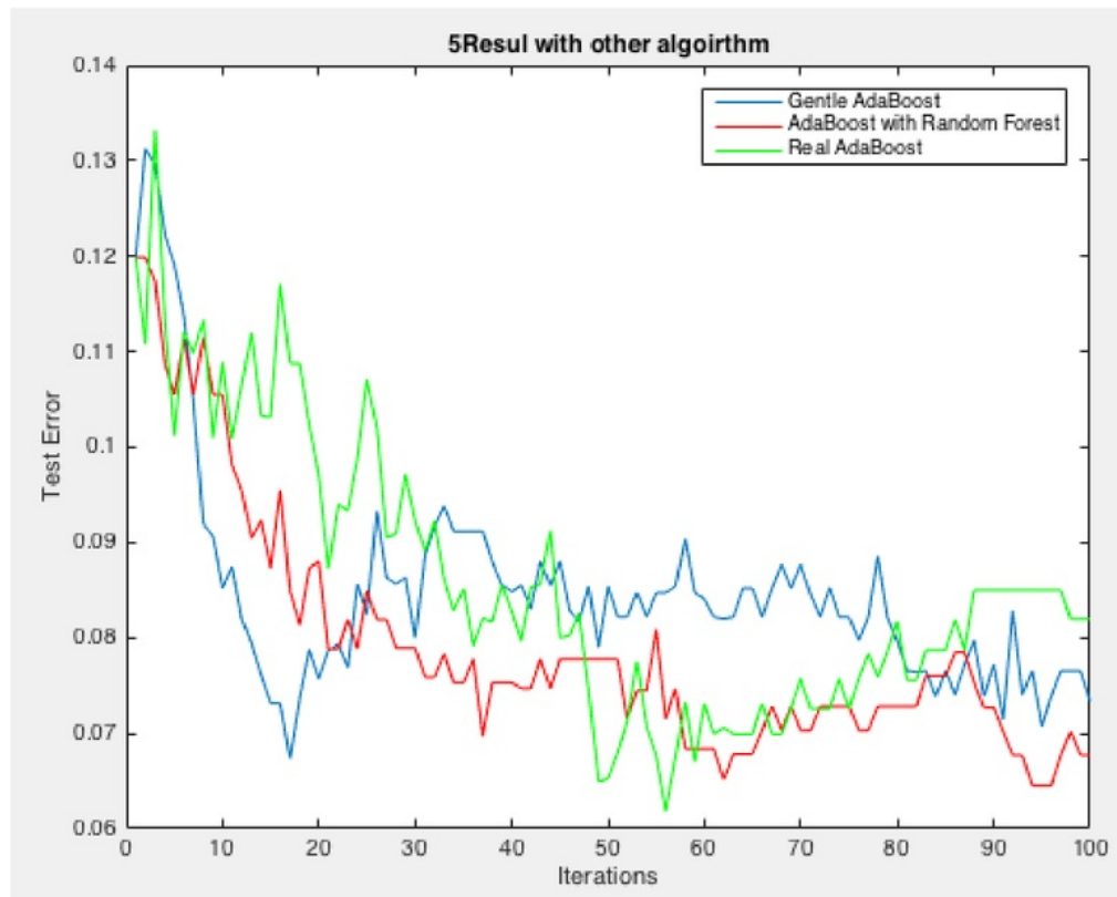
Gambar 7. Eksperimen 4.4.3 : Perbandingan hasil Algoritma
