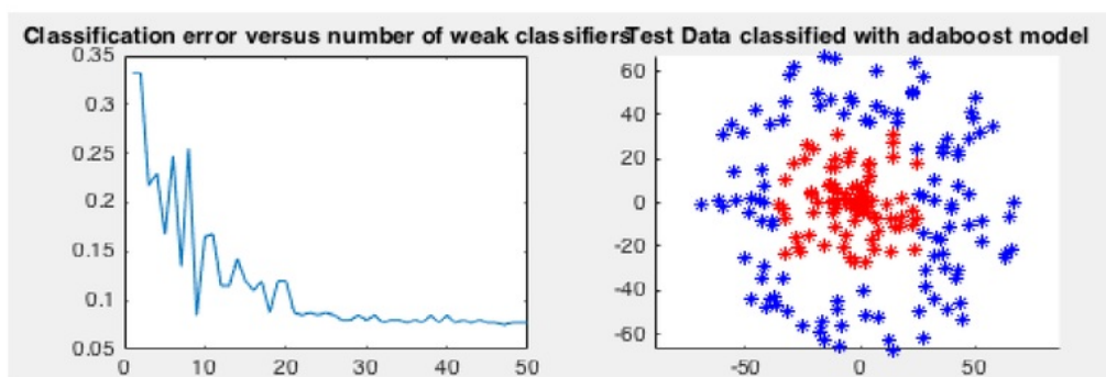
Gambar 8. Eksperimen 4.4.4 : Error h_1
