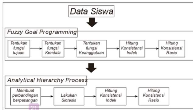
Gambar 2. Tahapan Penelitian
