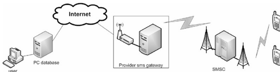
Gambar 1. Arsitektur Sistem Reminder
